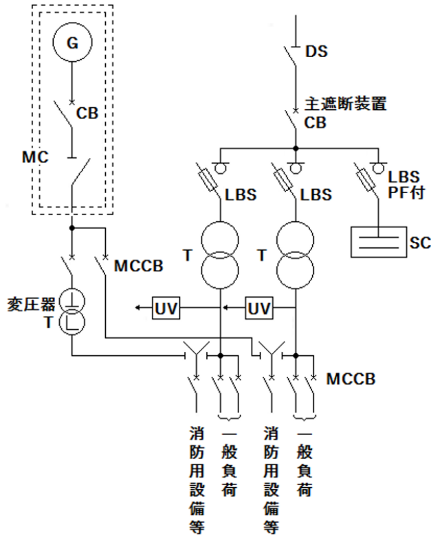
第3-13図 低圧自家発電設備の例
