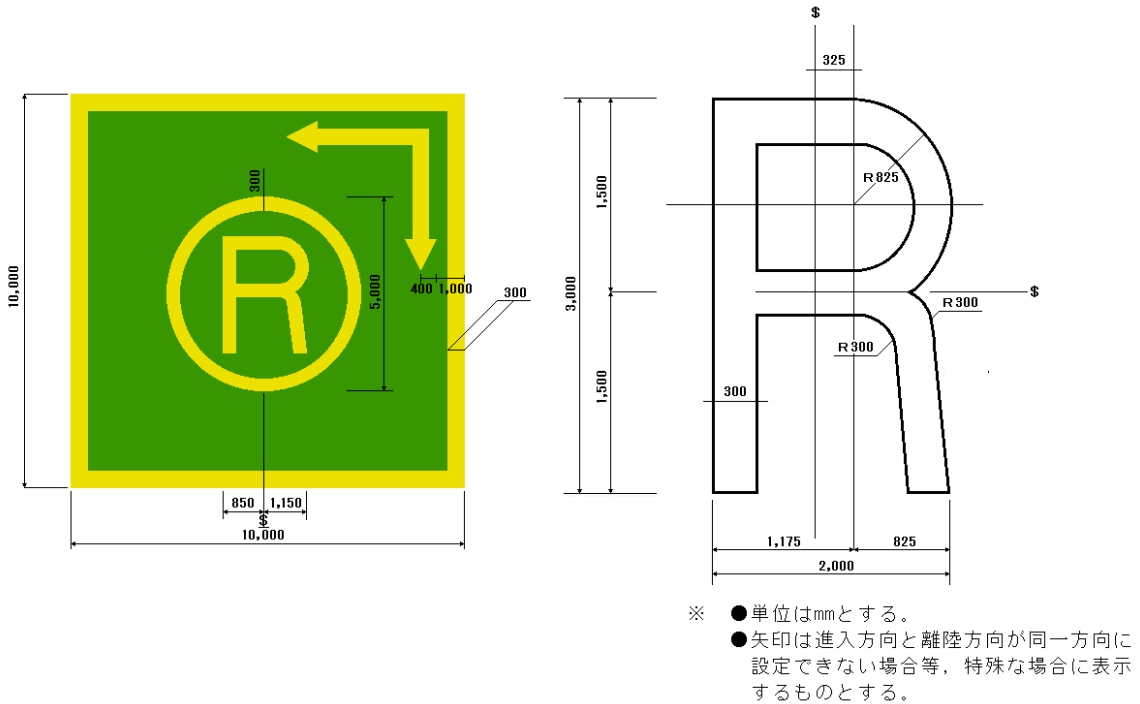
別図第12-2 緊急救助用スペース
