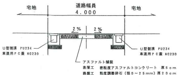
道路横断面図 A-A S1:100
