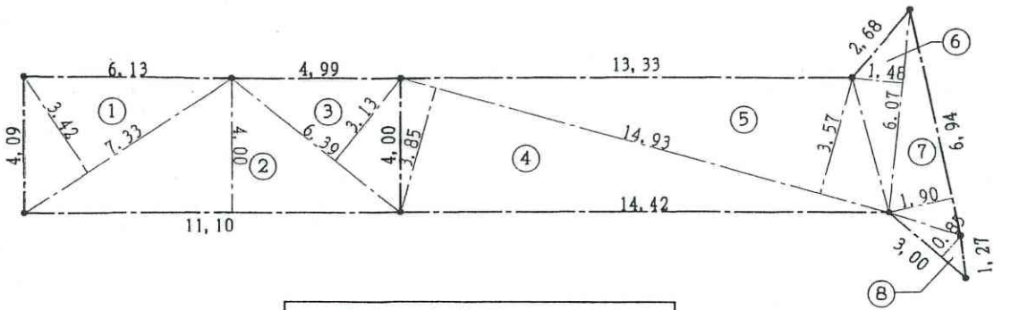
道路 求積図 S1:200
