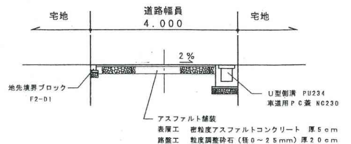
道路横断面図 B-B S1:100
