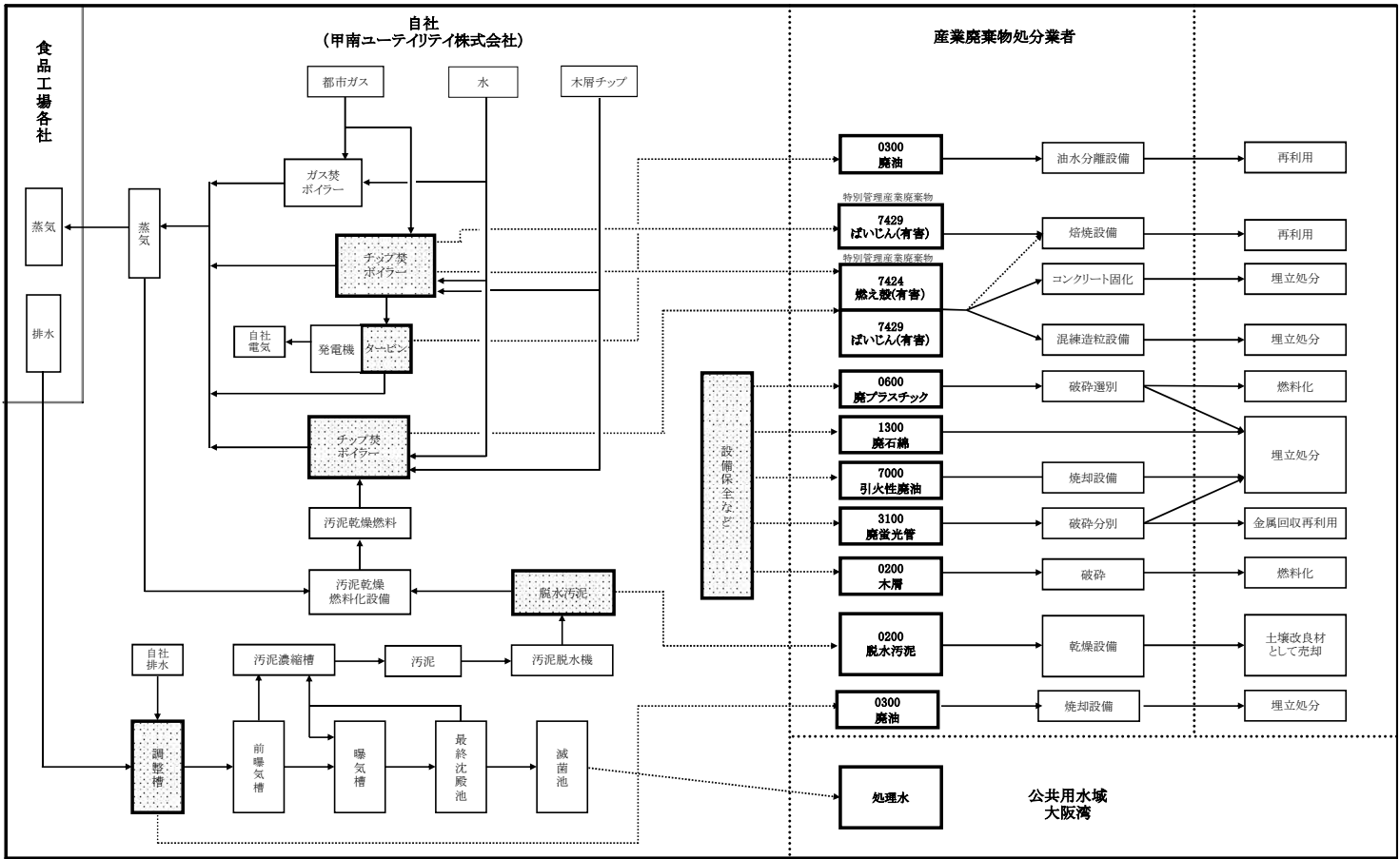
図1 産業廃棄物の一連の処理の工程
