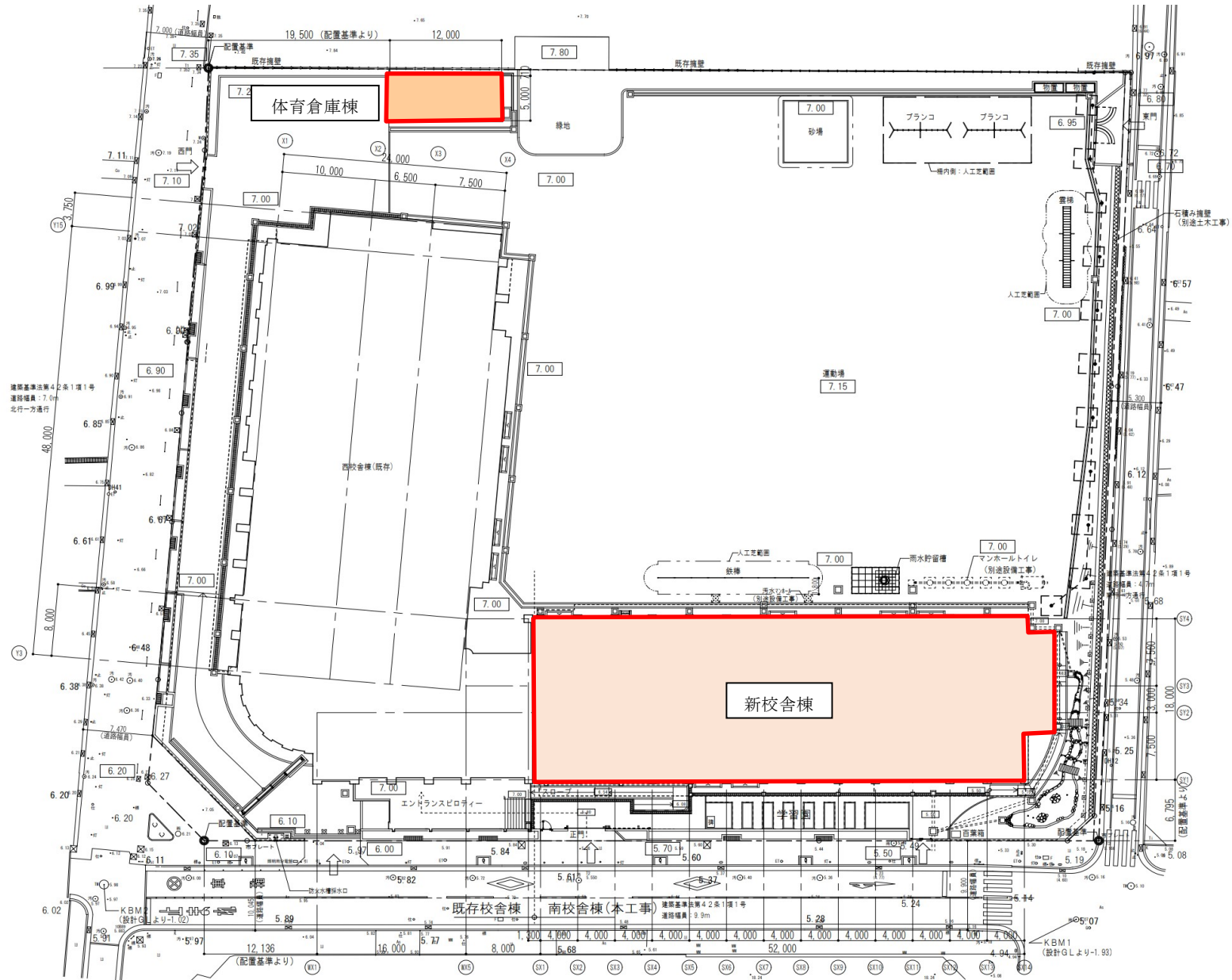
配置図
