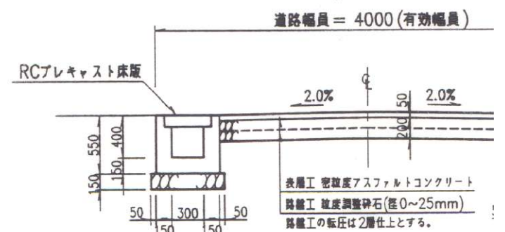
道路横断面図 S=1:
