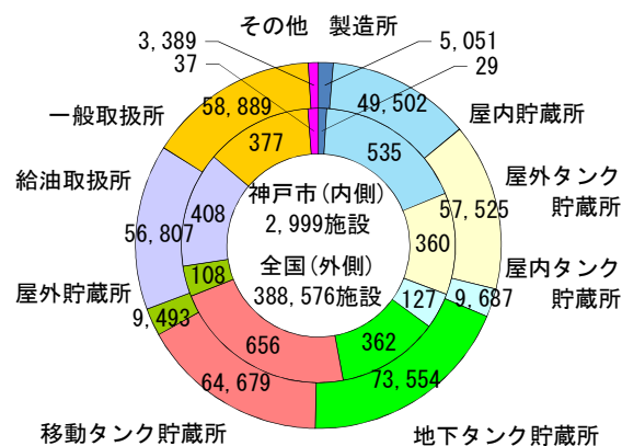
図5-1 危険物施設数区分別構成比
