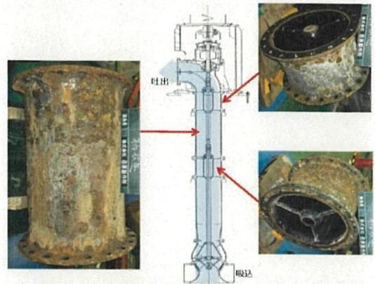
汚水ポンプの劣化状況 (経過年数 17 年 : 耐用年数 15 年)
