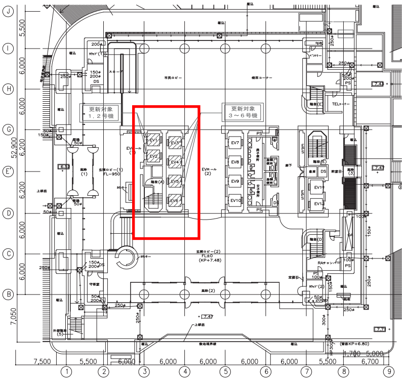
1号館1階平面図 1/200
