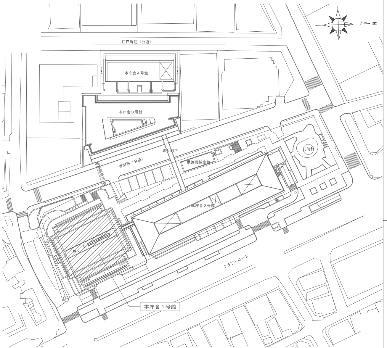
配置図 1/1,000
