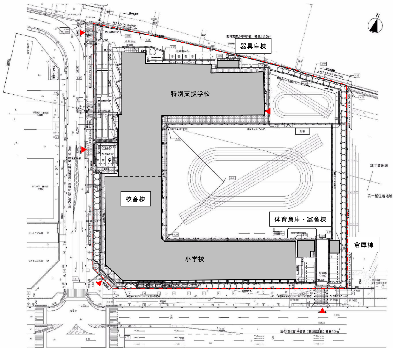
配置図
