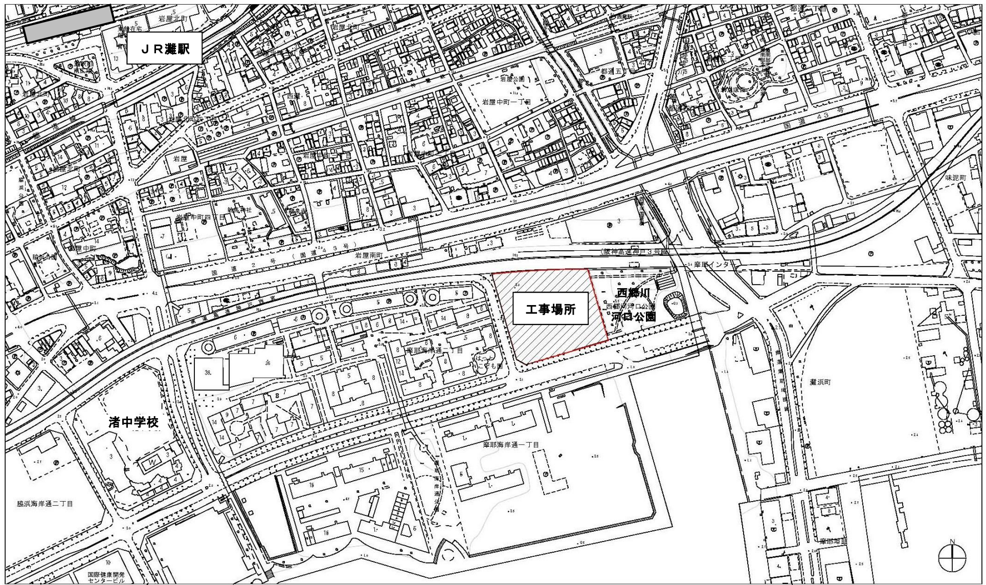
付近見取図
