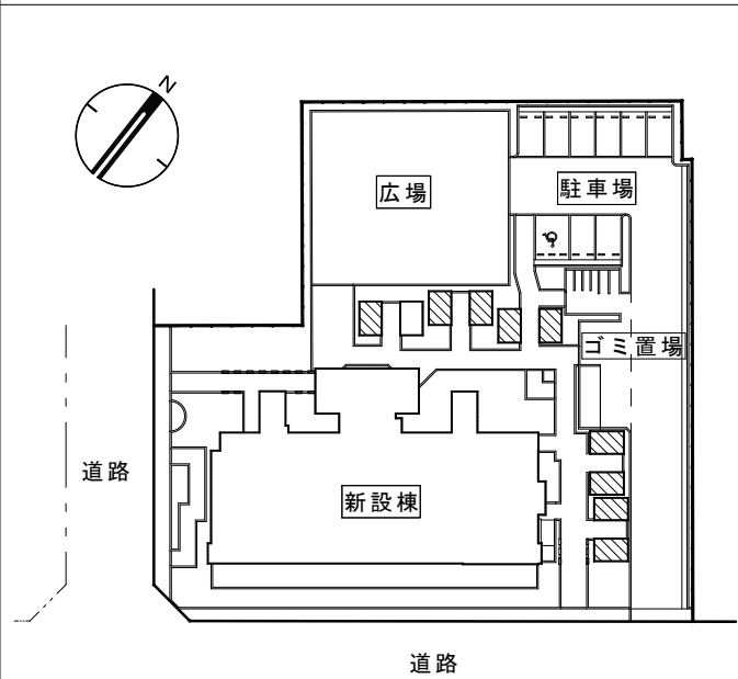
② 建築主体工 (1号棟跡地に新棟を建設)
